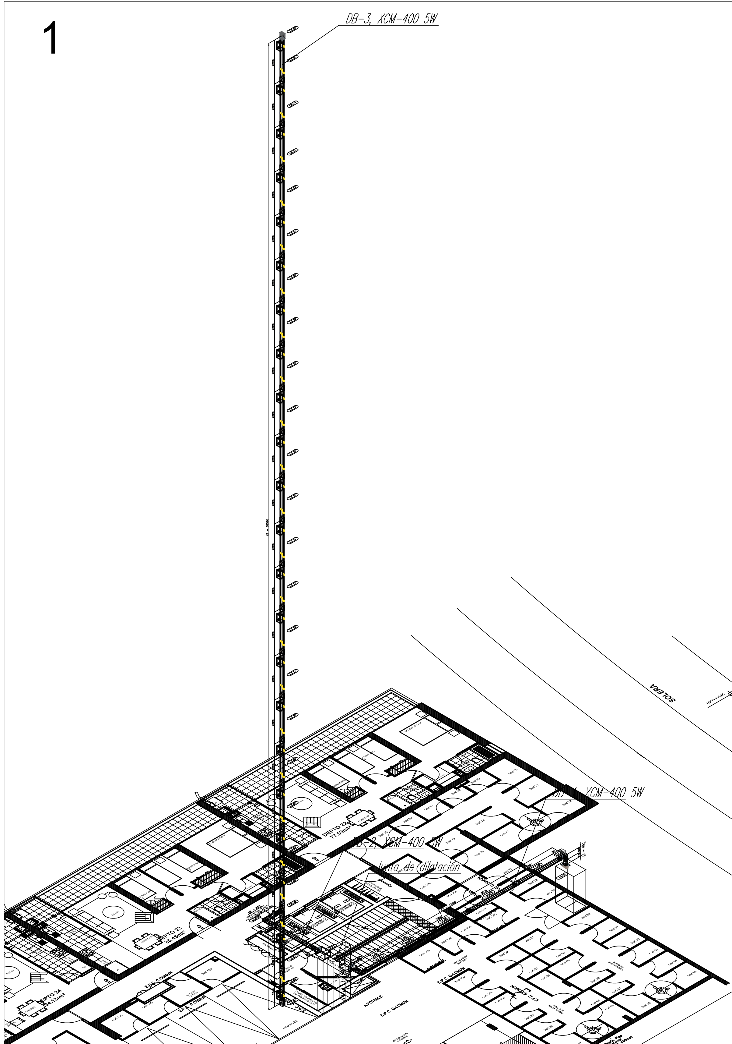
Vista isométrica estudio ducto barra.
